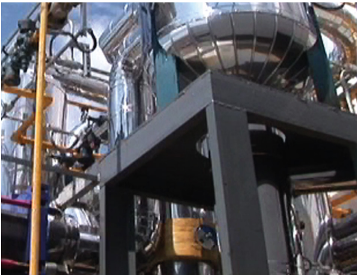
Unidad Productora de Hielo "Ice Maker Machine"
